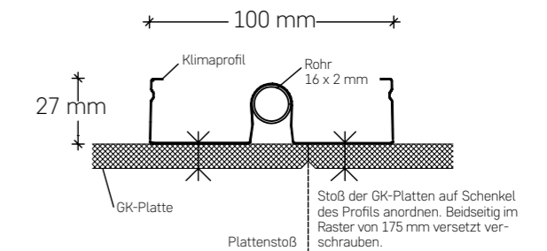
Verschraubung GK-Platte auf Klimaprofil
