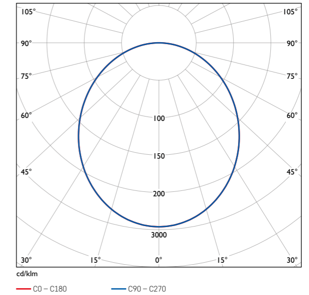
Lichtverteilungskurve Opal
