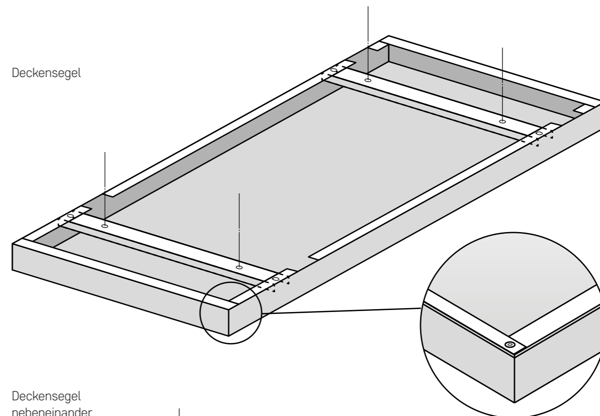
Rückseitige Umkantung wahlweise genietet
