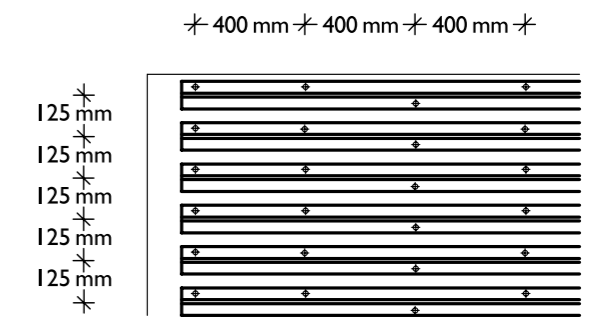
Verschraubungsschema (Achsabstand 125 mm)
