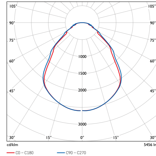
Lichtverteilungskurve Mikroprismen
